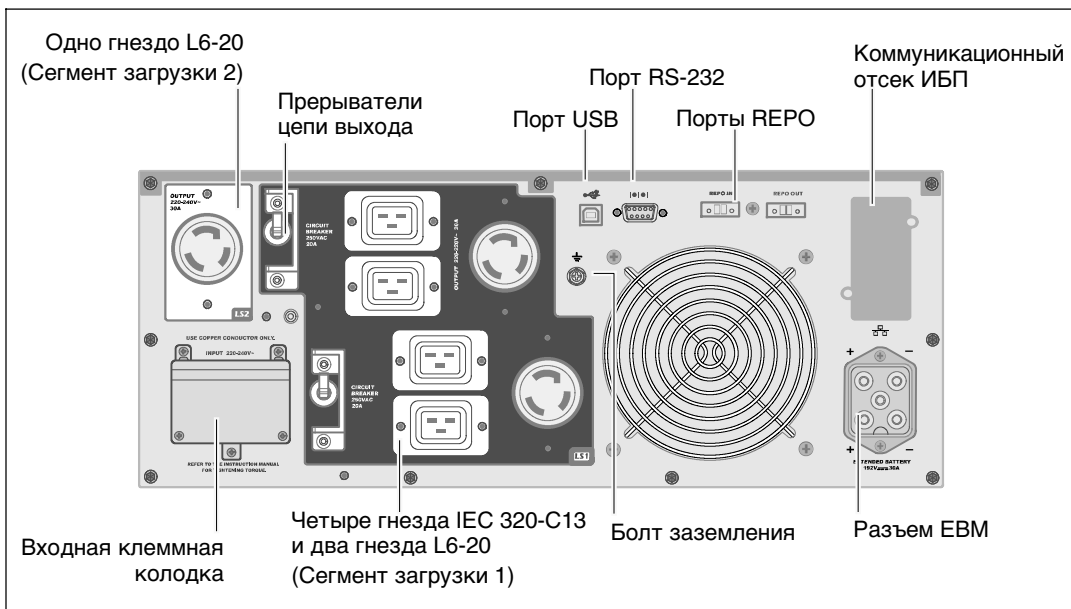
Рис. 7. 4200Вт, 208В задняя панель
