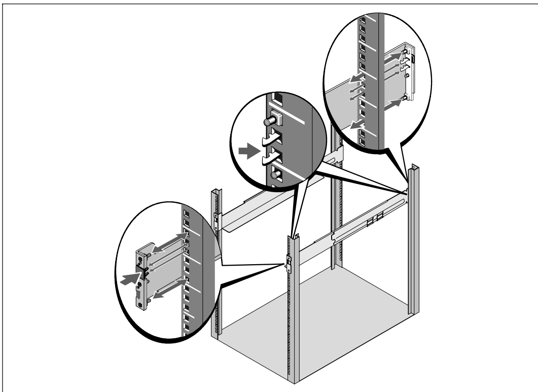
Рис. 12. Установка направляющих
