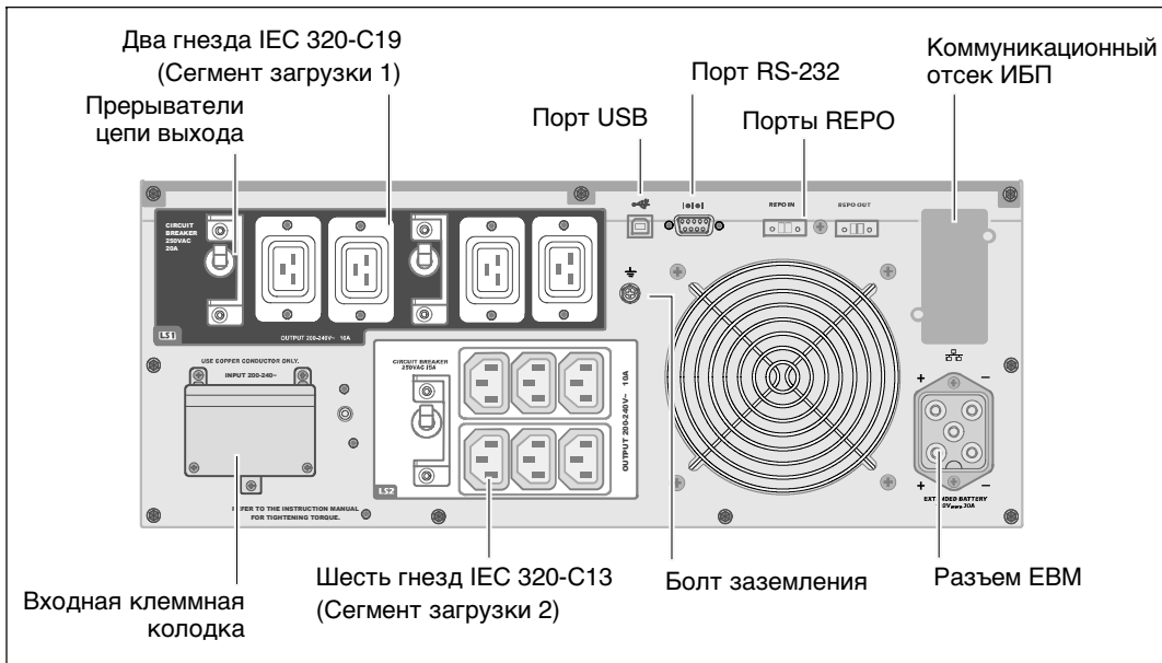
Рис. 6. 4200Вт, 200В задняя панель
