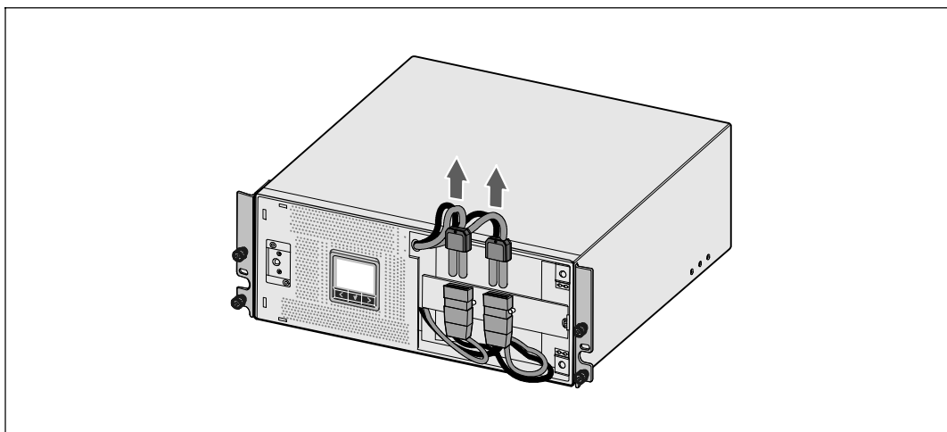
Рис. 28. Отсоединение внутреннего соединителя батареи
