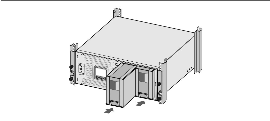
Рис. 15. Установите подставки для батарей
