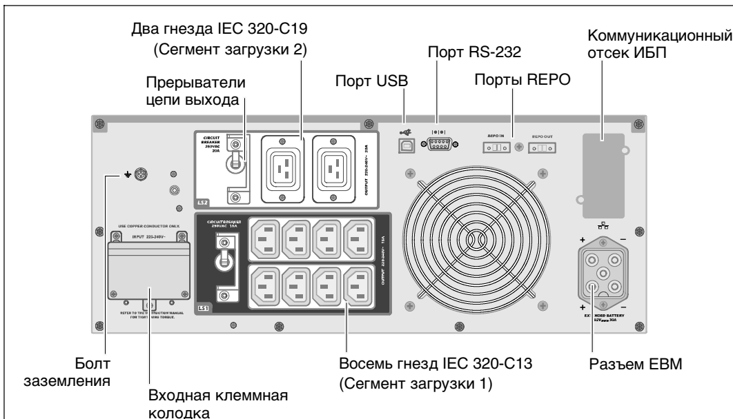
Рис. 5. 3750Вт, 230В Задняя панель
