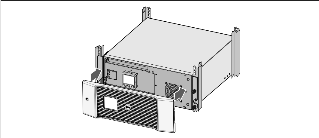
Рис. 17. Установка передней крышки ИБП
