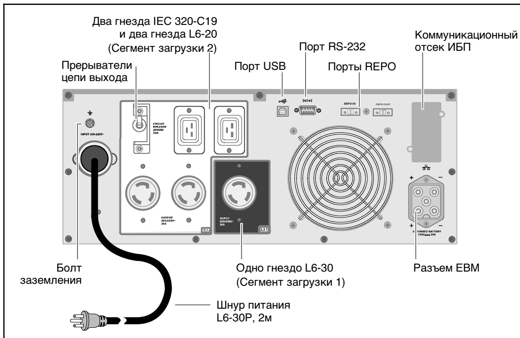
Рис. 4. 3750Вт, 208В Задняя панель
