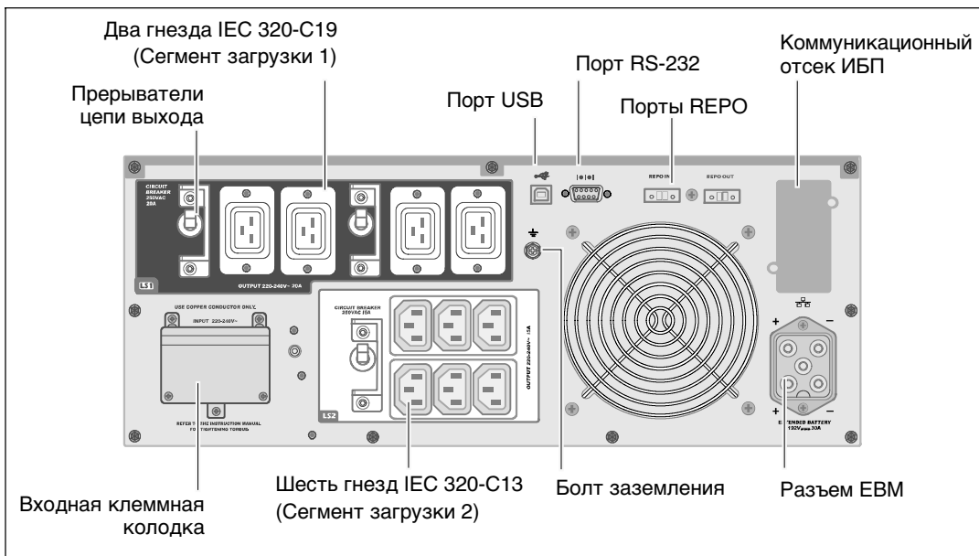
Рис. 8. 4200Вт, 230В задняя панель
