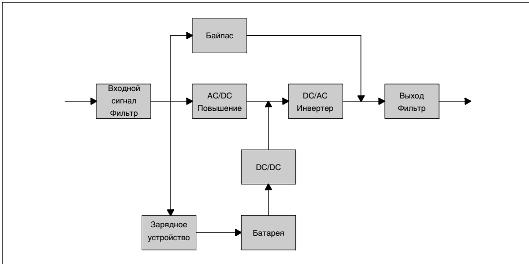
Рис. 30. Блок-схема онлайн для ИБП
