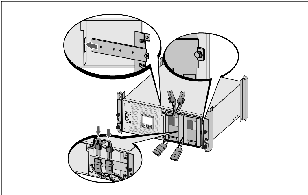
Рис. 16. Замена кронштейна, держащего батарею и подключение разъемов внешней батареи
