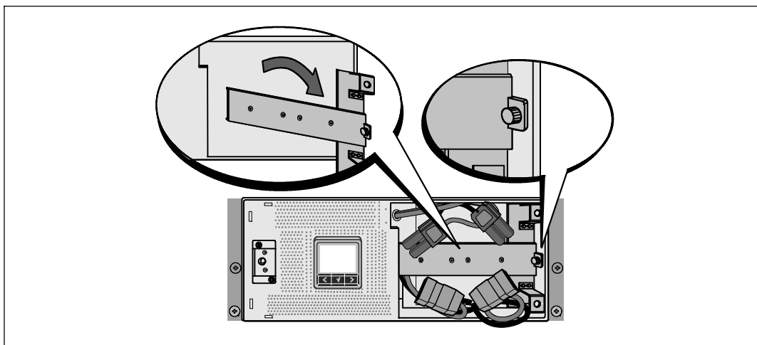
Рис. 10. Удаление кронштейна, держащего батарею
